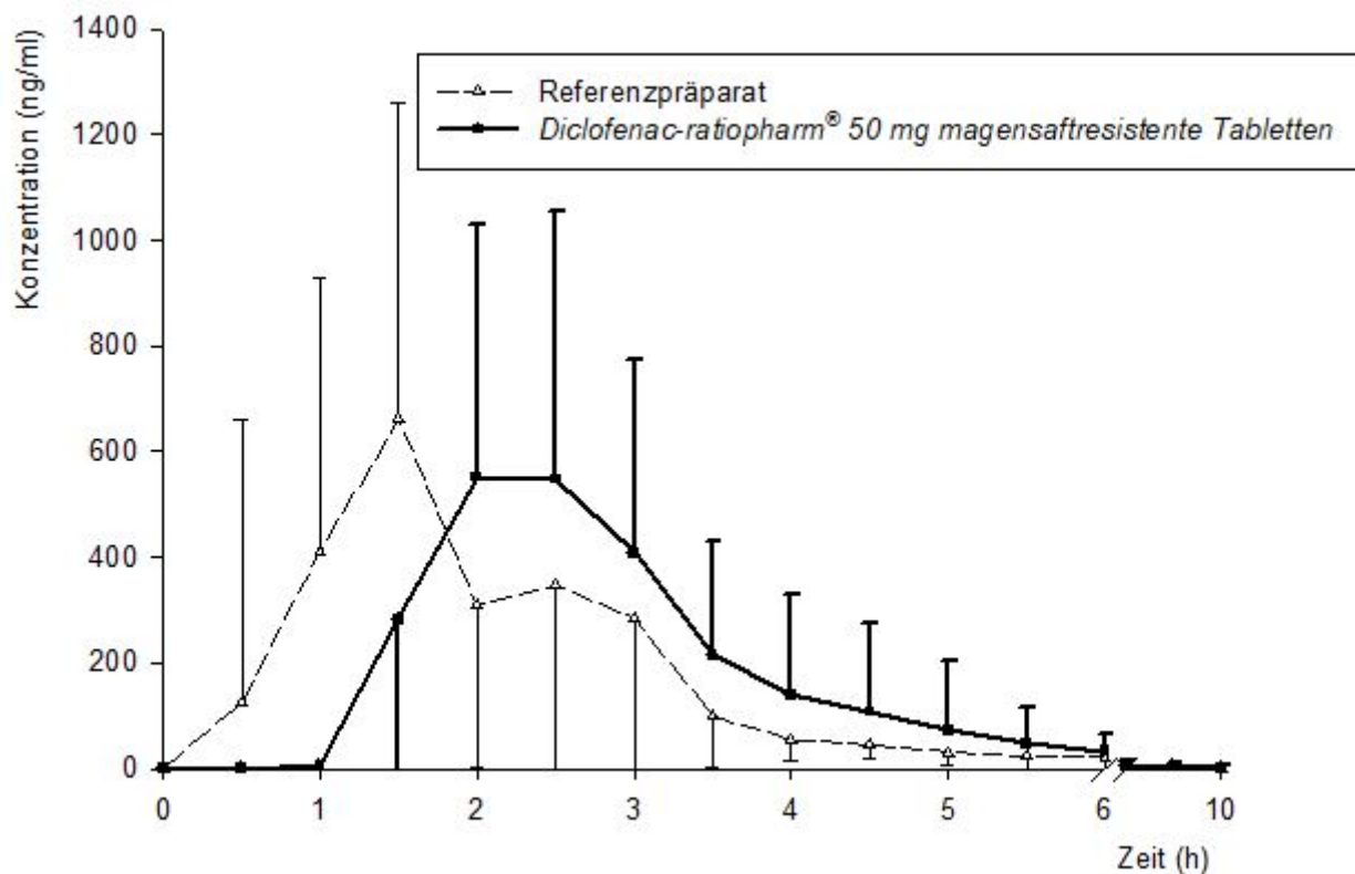
Abb. 2: Arithmetische Mittelwerte und Standardabweichungen der Plasmakonzentration von Diclofenac nach Einmalgabe von 1 magensaftresistenten Tablette Diclofenac-ratiopharm ® 50 mg magensaftresistente Tabletten bzw. 1 magensaftresistenten Tablette Referenzpräparat.
