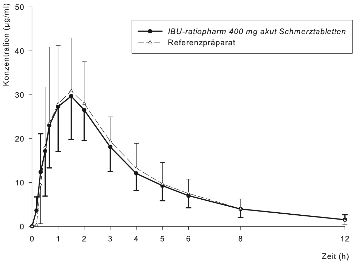
Abb. 2: Mittelwerte und Standardabweichungen der Plasmakonzentration von Ibuprofen nach Einmalgabe von 1 Filmtablette IBU-ratiopharm 400 mg akut Schmerztabletten bzw. 1 Dragee Referenzpräparat.
