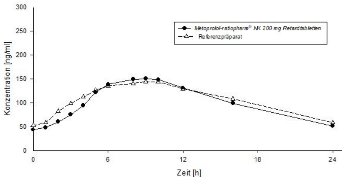
Abb. 2: Mittelwerte und Standardabweichungen der Plasmakonzentration von Metoprolol nach siebenmaliger täglicher Einmalgabe von 1 Retardtablette Metoprolol-ratiopharm® NK 200 mg Retardtabletten bzw. Referenzpräparat
