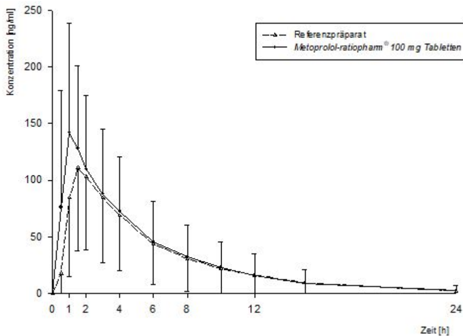
Abb. 1: Mittelwerte und Standardabweichungen der Plasmakonzentration von Metoprolol nach Einmalgabe von 1 Tablette Metoprolol-ratiopharm® 100 mg Tabletten bzw. Referenzpräparat.
