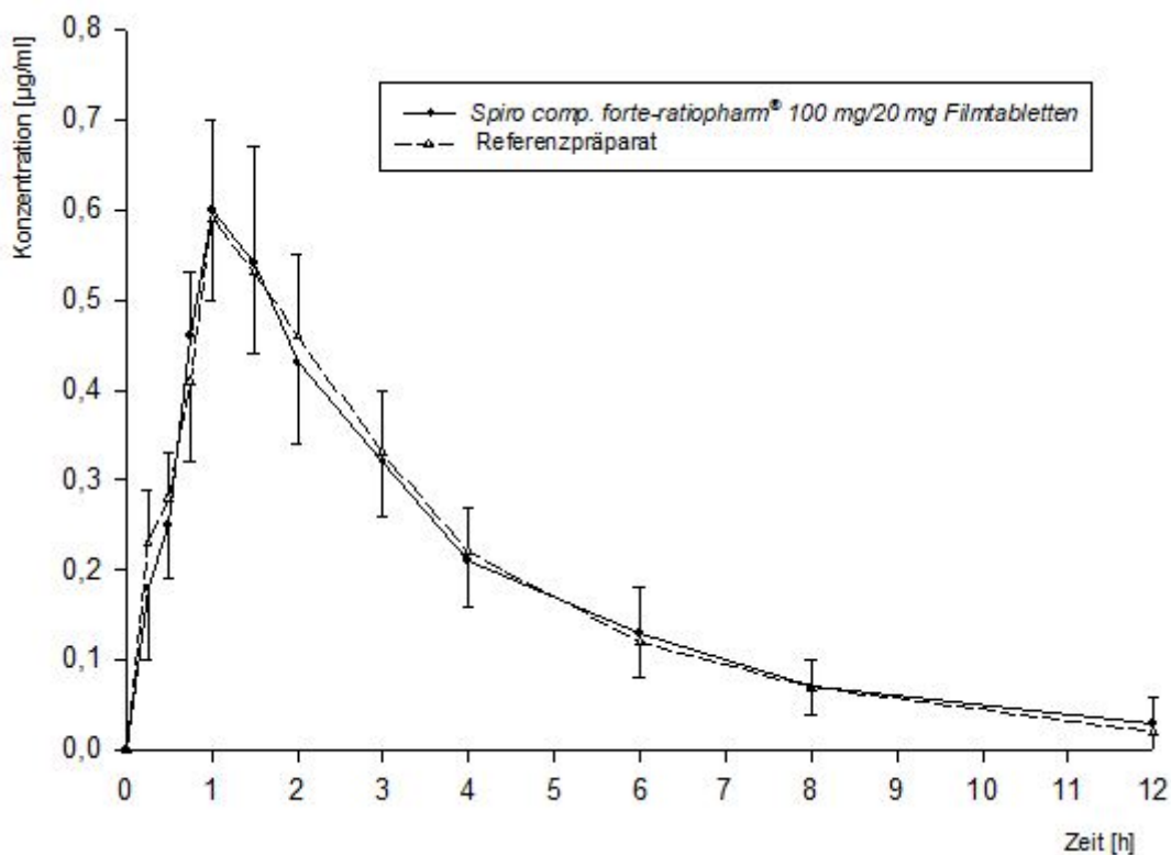
Abb. 1: Mittelwerte und Standardabweichungen der Plasmakonzentration von Furosemid nach Einmalgabe von 1 Tablette Spiro comp. forte-ratiopharm® 100 mg/20 mg Filmdabletten bzw. Referenzpräparat.
