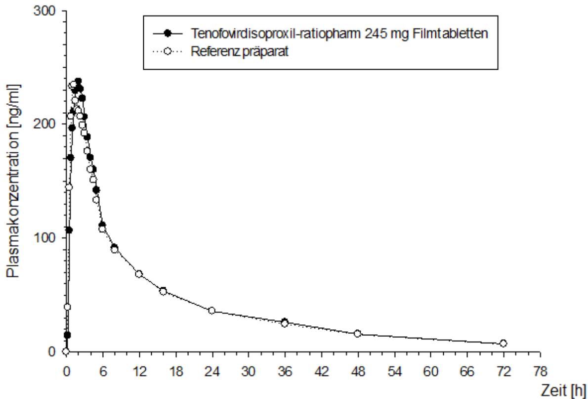
Abb.: Mittelwerte der Plasmakonzentration von Tenofoviridisoproxil nach Einmalgabe von 1 Filmtablette Tenofoviridisoproxil-ratiopharm ® 245 mg Filmtabletten bzw. Referenzpräparat (Viread ® ).
